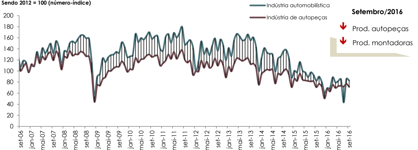
[Gráfico 6] Produção industrial das autopeças x das montadoras
